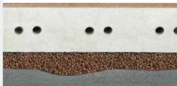
Betonový strop s mokřím potěrem
